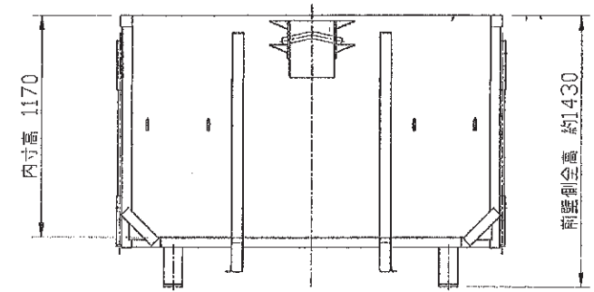
A 矢視図
